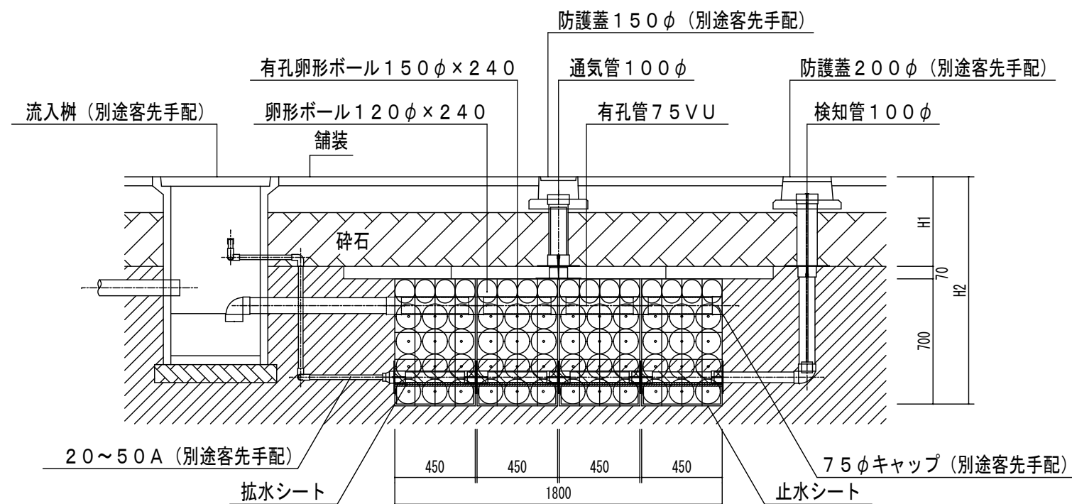
A-A断面図
