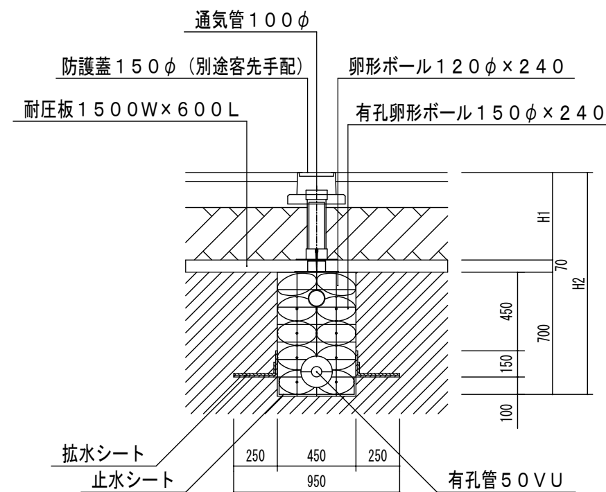
B-B断面図
