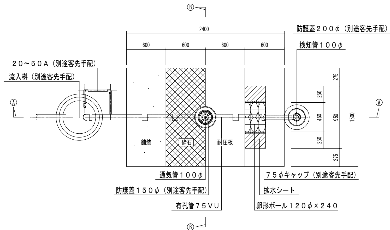
SRS-EPS土壌拡散処理システム平面図
