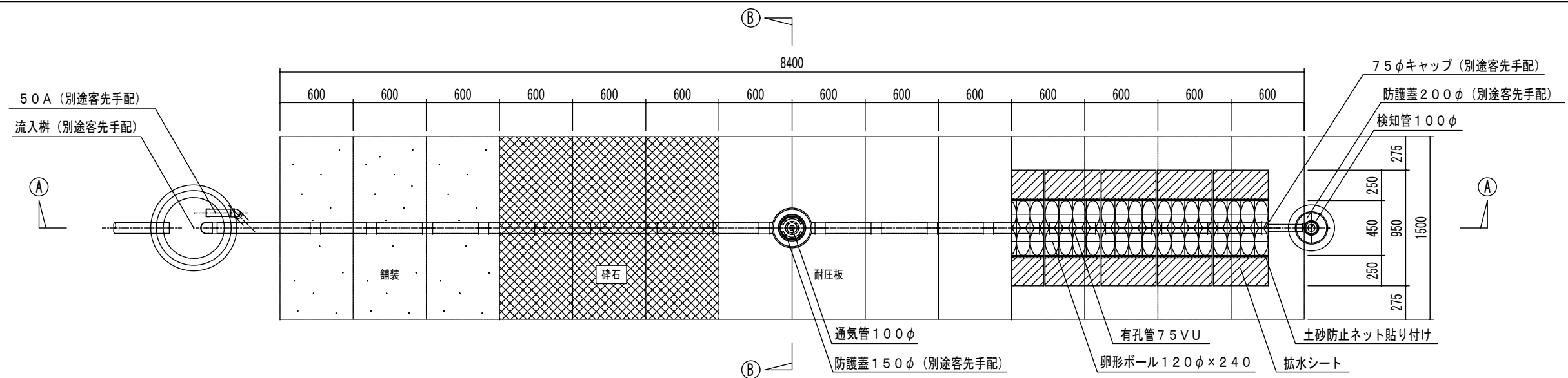
SRS-EPS土壌拡散処理システム平面図
