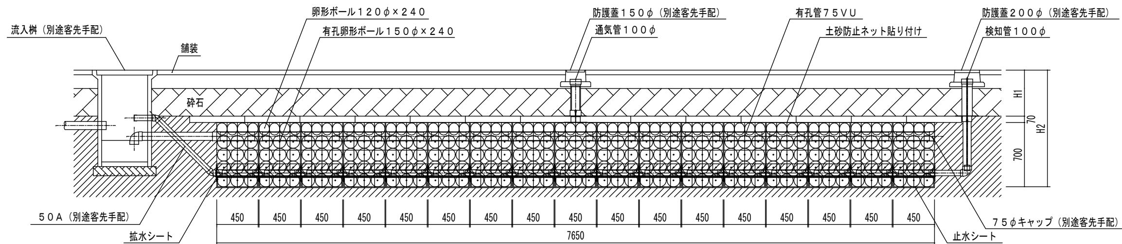
A-A断面図
