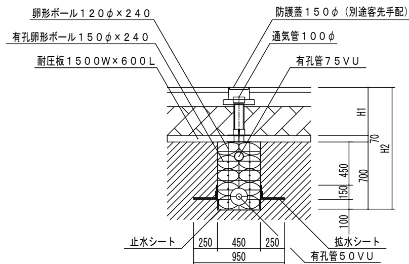
B-B断面図
