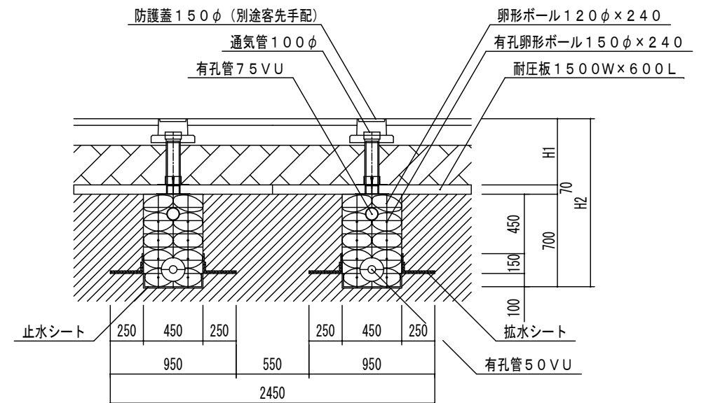
B-B断面図
